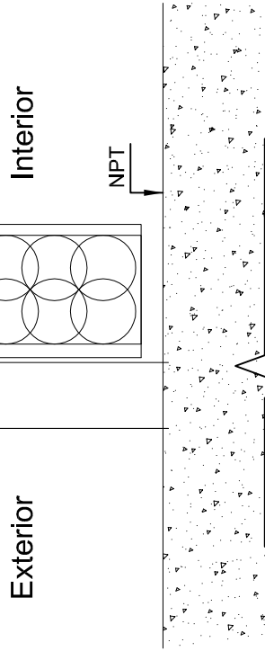
CORTE 2-2 - Esc.: 1:2.5
