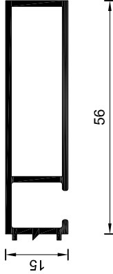
Tipo MT-6517 Premarco Peso estimado: 0.532 Kg/m Largo STD: 6200mm
