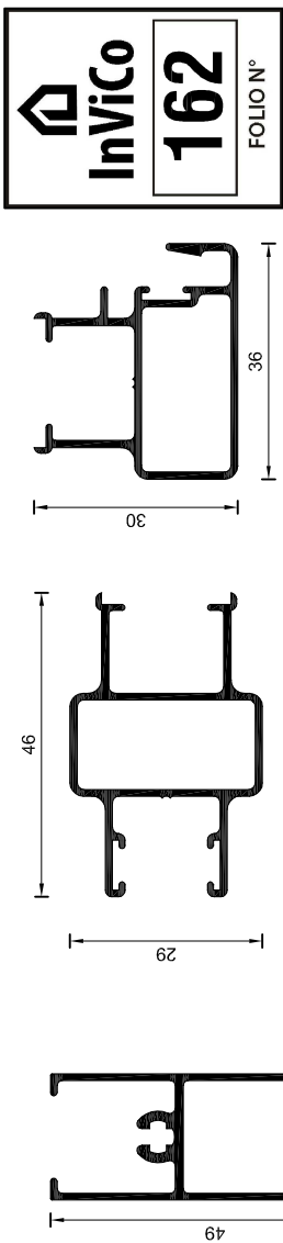
Tipo MT-0903 Parante lateral hoja corrediza Peso estimado: 0.462 Kg/m Largo STD: 6150 mm
