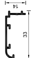
Tipo MT-0829 Contramarco Peso estimado: 0.197 Kg/m Largo STD: 6030 mm
