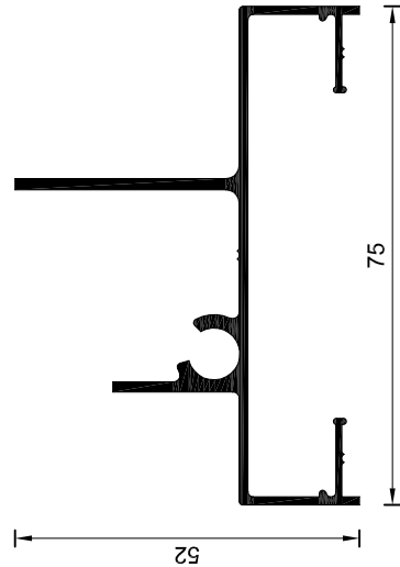
Tipo MT-0916 Marco ventana proyectante o banderola Peso estimado: 0.716 Kg/m Largo STD: 6150 mm
