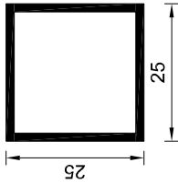
TC-025 Tipo cuadrado Peso estimado: 0.381 Kg/m
