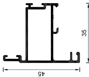
Tipo MT-0915 Bisagra vent. proyectante o banderola Peso estimado: 0.281 Kg/m Largo STD: 6030 mm
