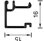
Tipo MT-0908 Contravidrio universal Peso estimado: 0.151 Kg/m Largo STD: 6030 mm
