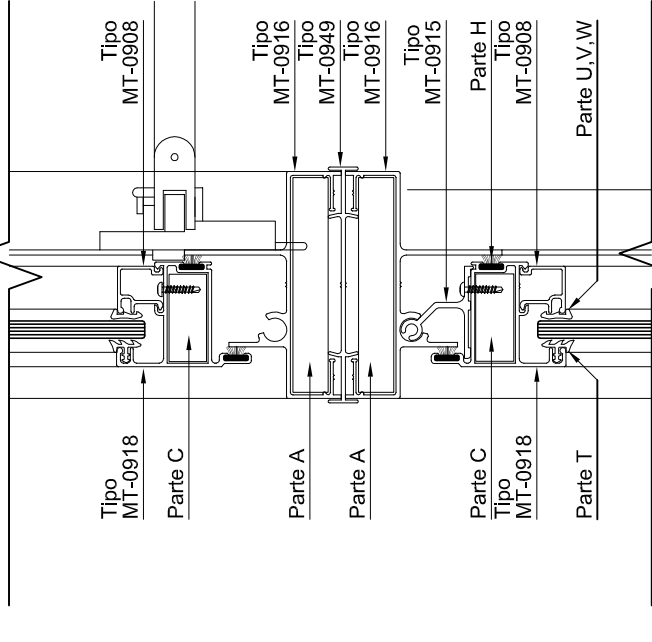
CORTE 2-2 - Esc.: 1:2.5
