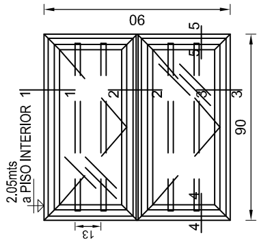
VISTA INTERIOR - Esc.: 1:25
