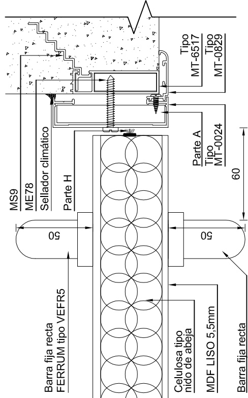
CORTE 4-4 - Esc.: 1:2.5
