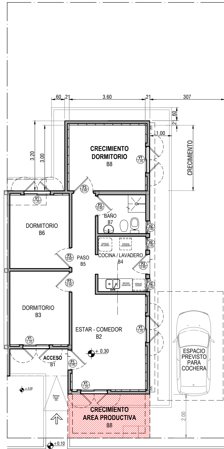
PLANTA - ESC: 1:100
