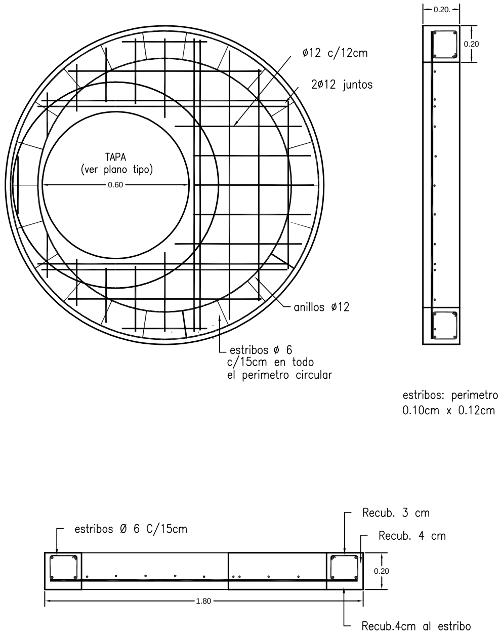
TAPA BOCA DE REGISTRO DETALLE LOSA Y TAPA DE H° A° PREFABRICADOS
