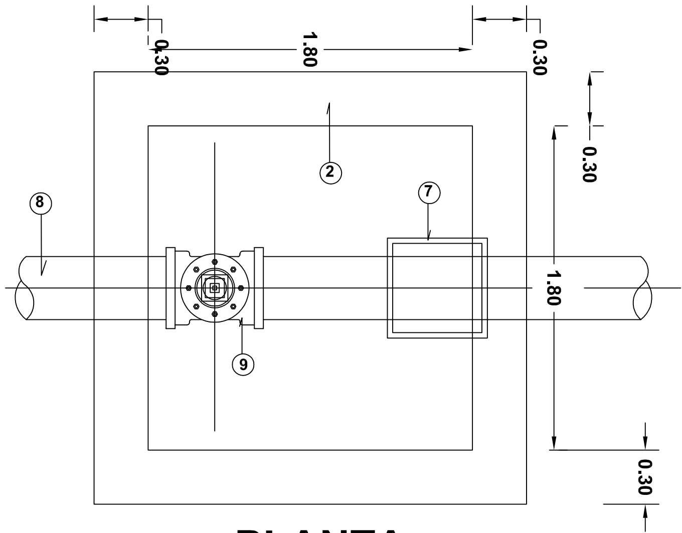
PLANTA
