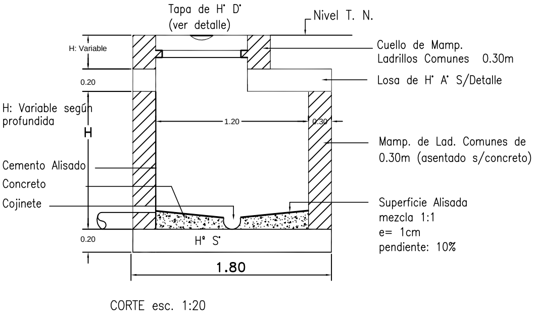
BOCA DE REGISTRO CON LOSA SUPERIOR Y TAPA DE H° A°
